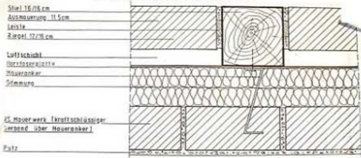
Horizontaler Schnitt
